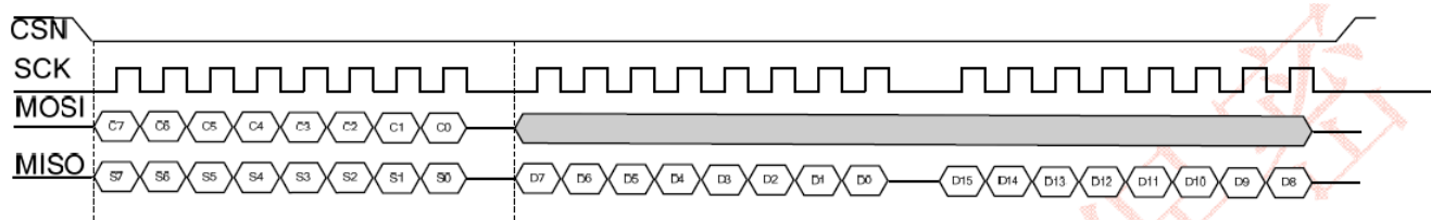
图 5-5 SPI 读操作时序图
