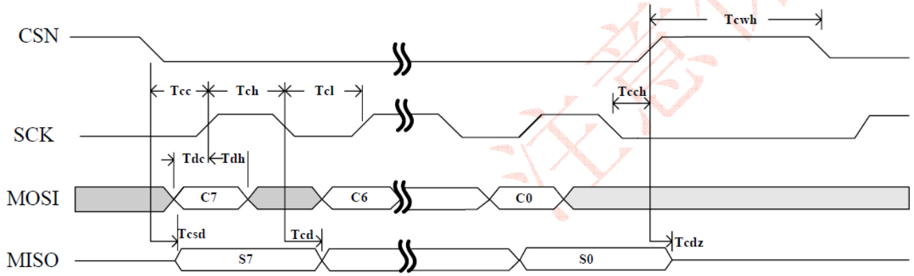
图 5-7 SPI 典型时序图
