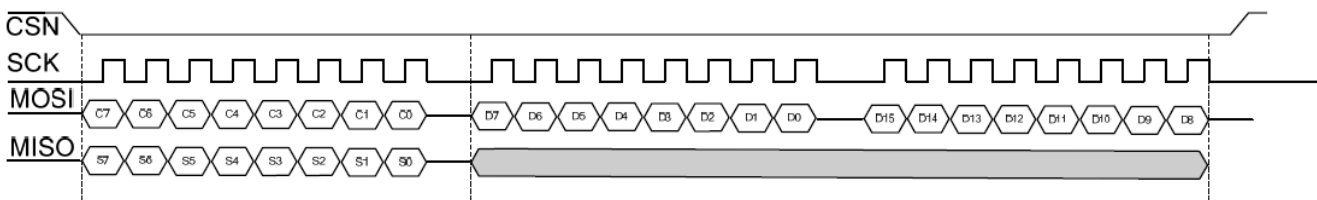
图 5-6 SPI 写操作时序图
