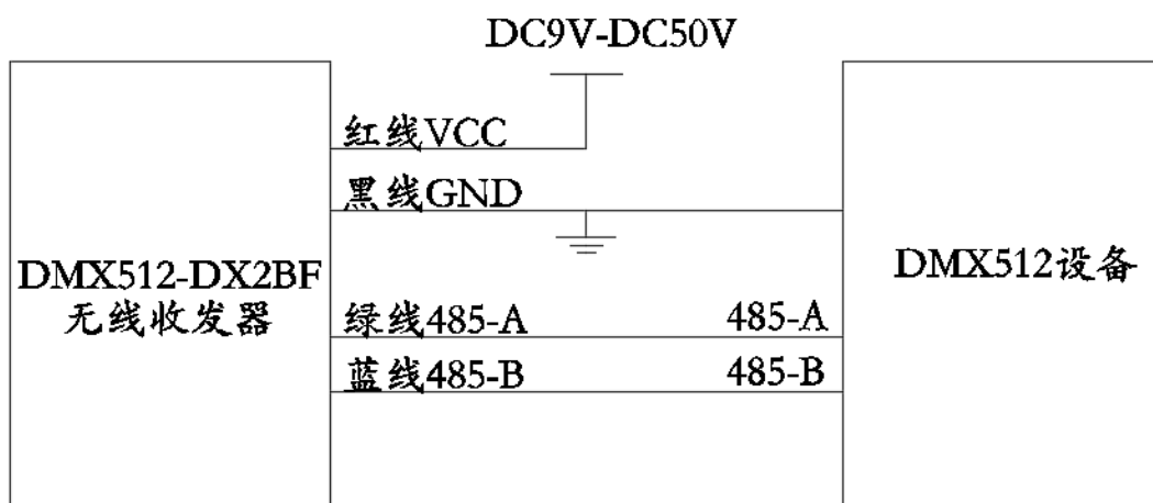
DMX512-DX2BF 接线示意图
