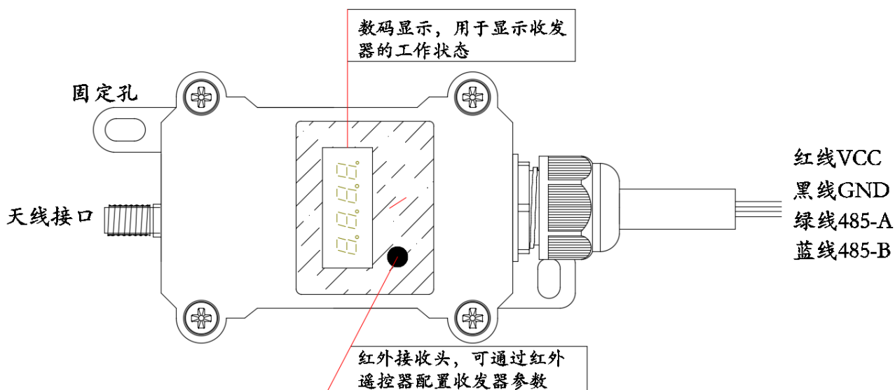
DMX512-DX2BF 产品示意图
