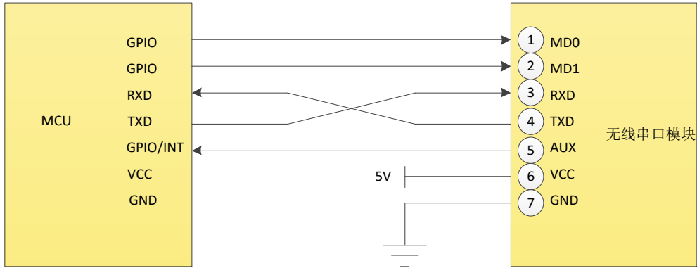
图 5-1 推荐连接图
