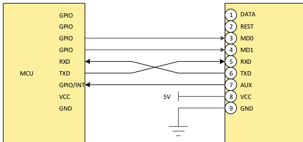
图 5-1 推荐连接图
