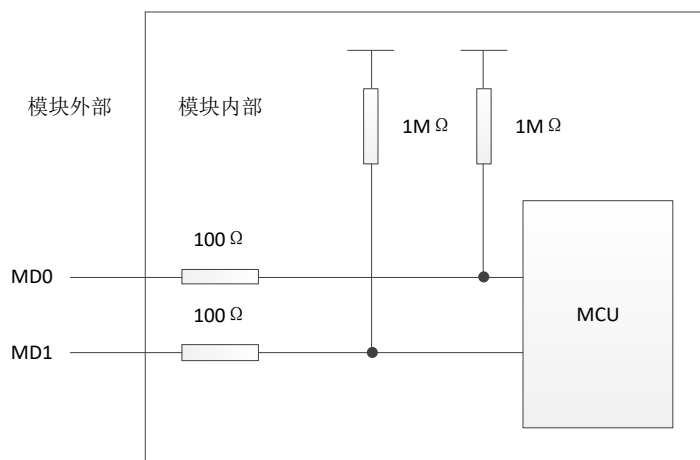
图 5-2 MD0、MD1 引脚内部结构示意图
