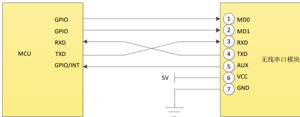
图 5-1 推荐连接图
