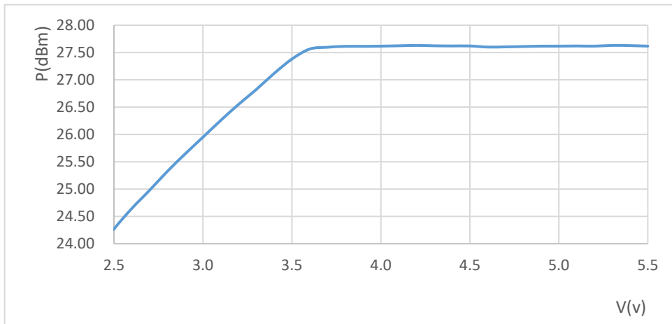
图 5-7 功率与电压的关系图
