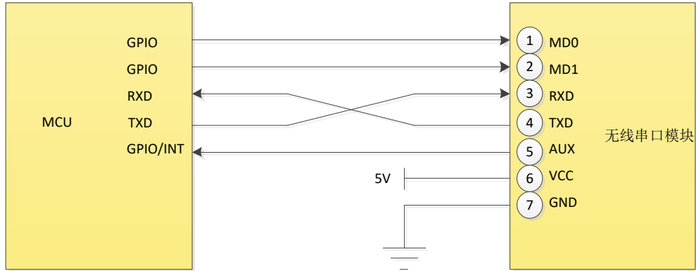
图 5-1 推荐连接图
