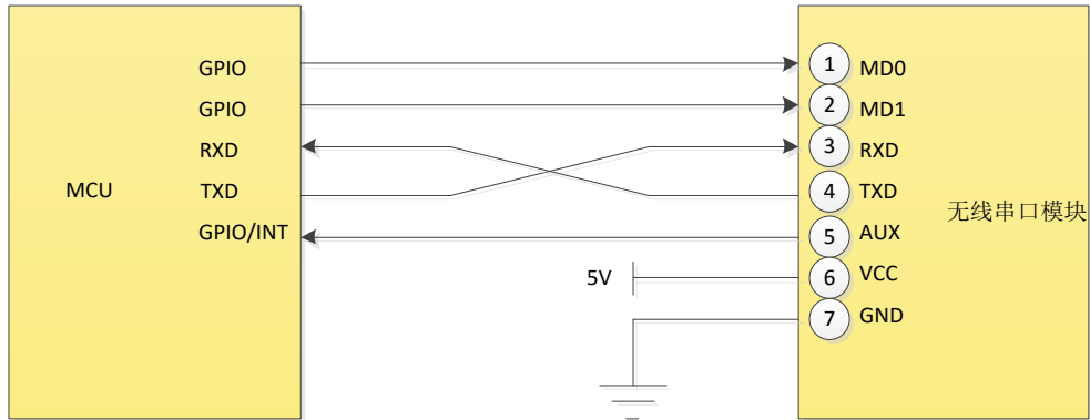
图 5-1 推荐连接图
