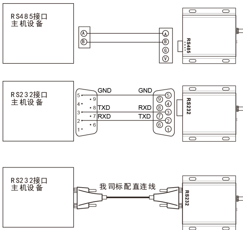
图 5-1 推荐连接图
