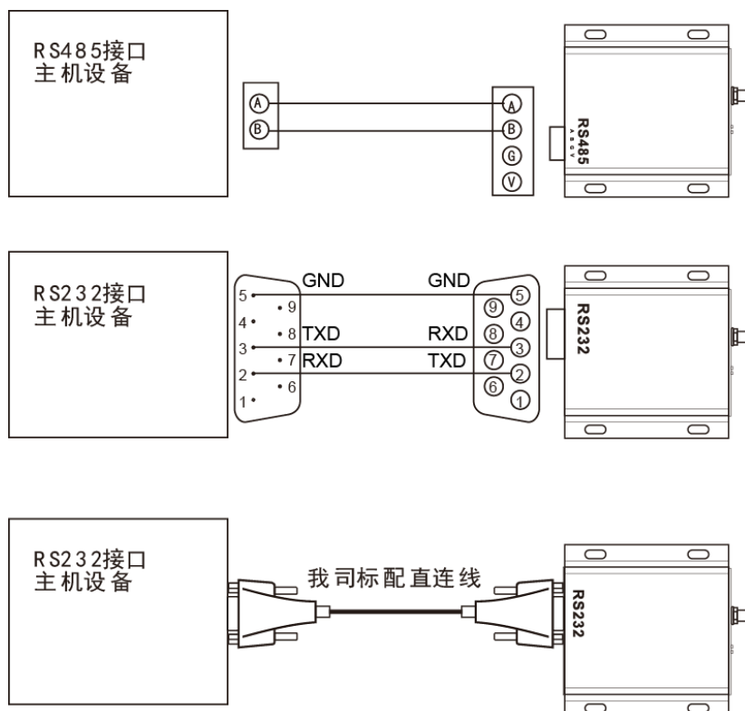
图 5-1 推荐连接图
