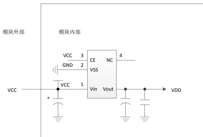
图 5-6 电源 LDO
