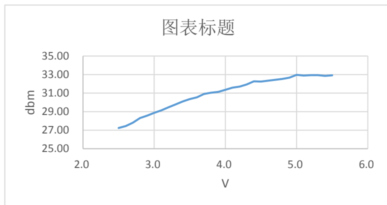
图 5-7 功率与电压的关系图
