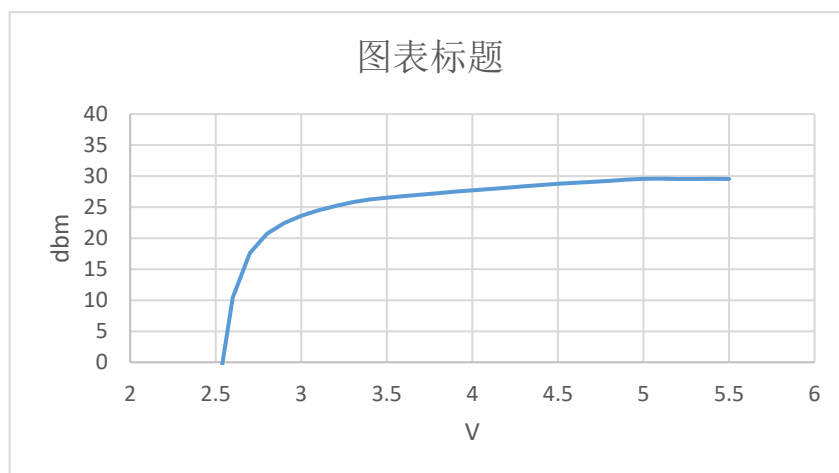
图 5-7 功率与电压的关系图
