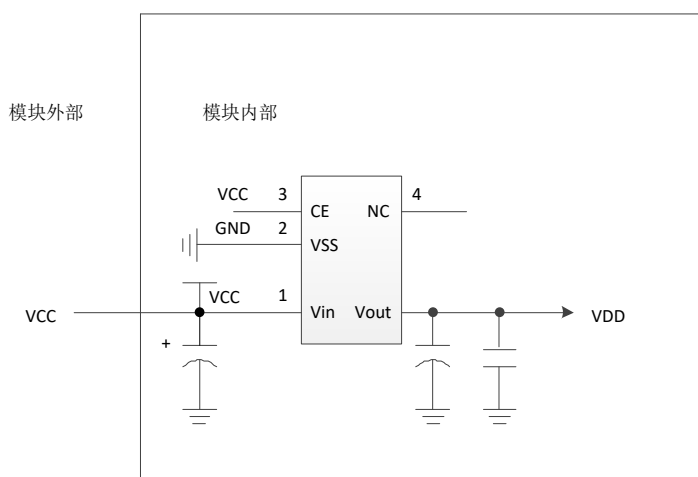
图 5-6 电源 LDO
