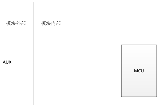
图 5-3 AUX 引脚内部结构示意图
