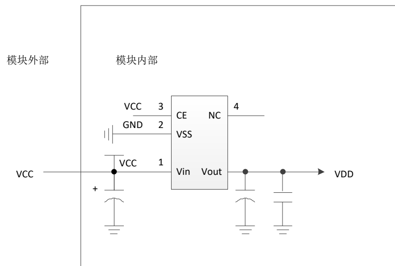
图 5-6 电源 LDO
