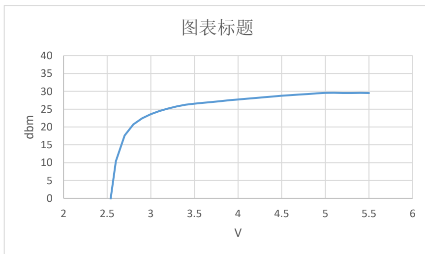
图 5-7 功率与电压的关系图
