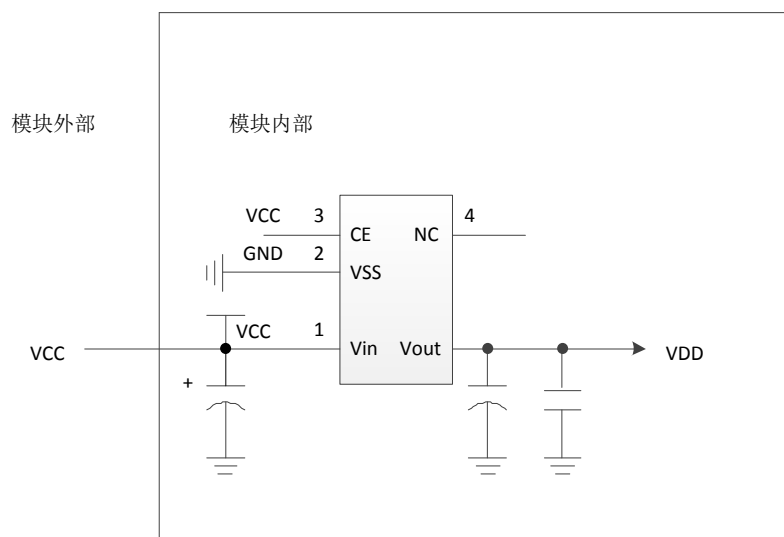
图 5-6 电源 LDO
