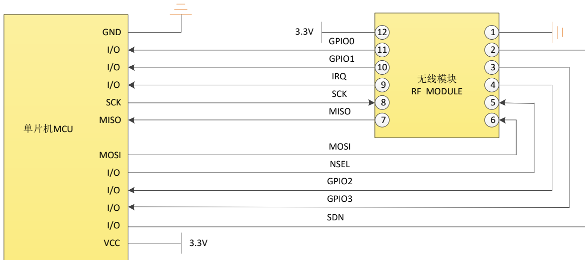
图 5-1 推荐连接图
