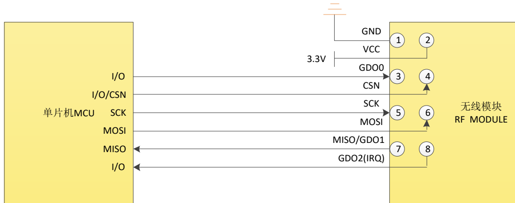
图 5-1 推荐连接图
