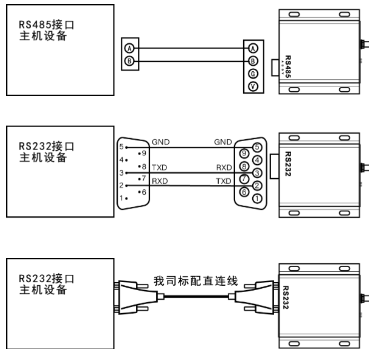
图 5-1 推荐连接图
