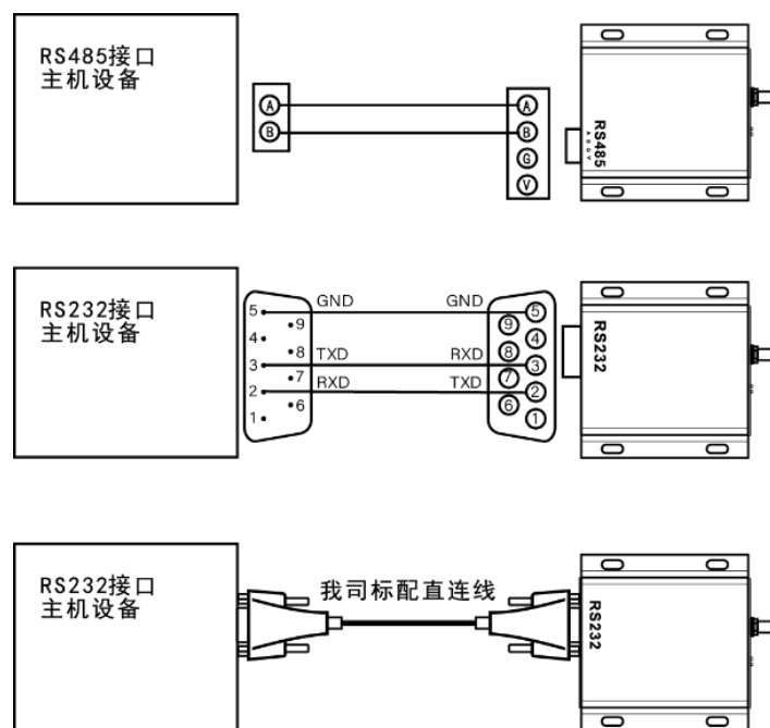
图 5-1 推荐连接图
