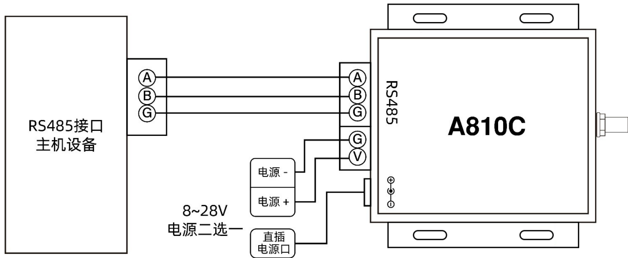
图 5-1 推荐连接图
