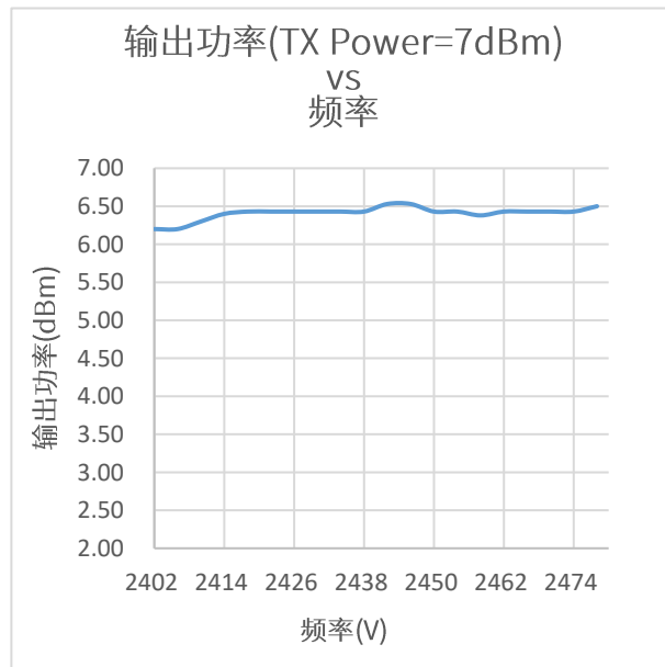
图 4-2 输出功率(TX Power=7dBm) vs 频率
