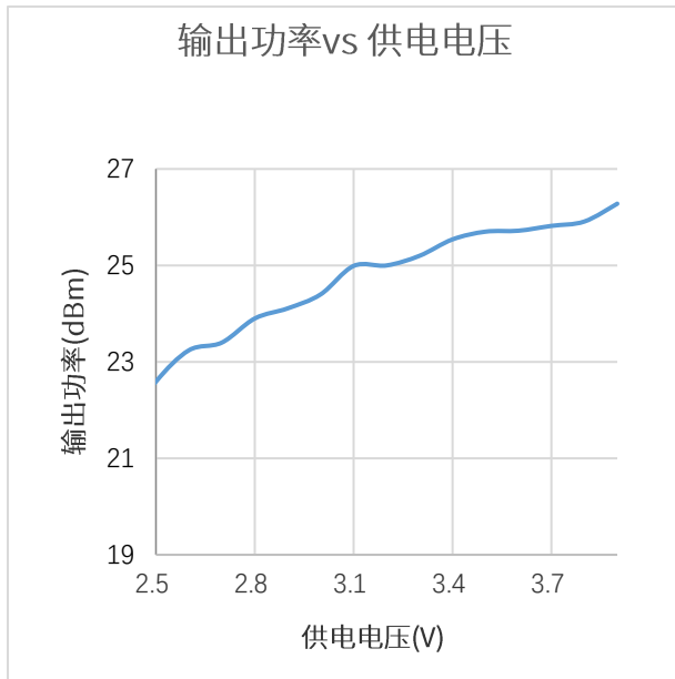
图 4-8 输出功率 vs 供电电压
