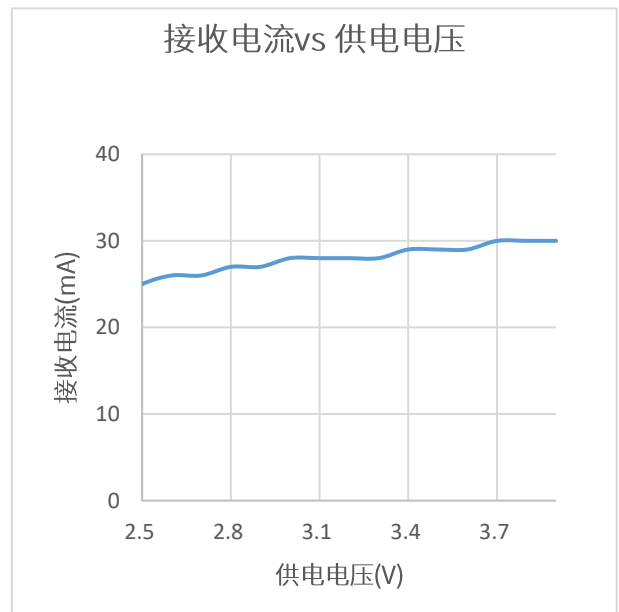
图 4-12 输出功率(输入功率-100dBm) vs 供电电压
