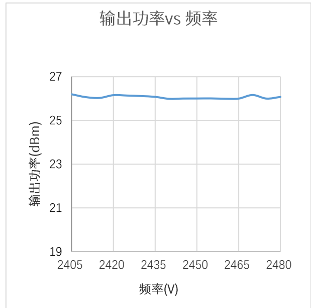
图 4-9 输出功率 vs 频率
