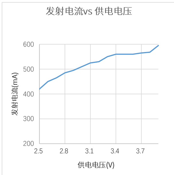
图 4-10 发射电流 vs 供电电压
