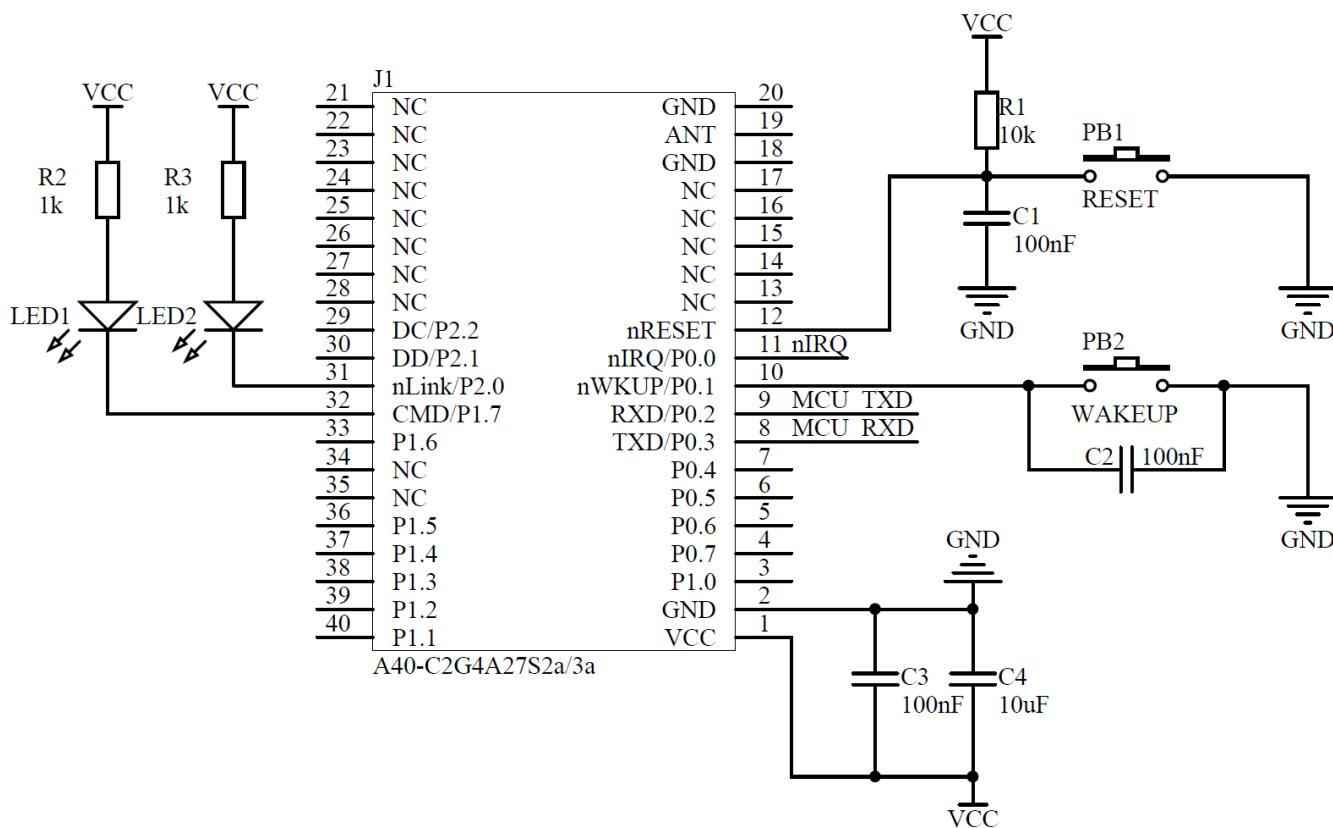
图 5-1 A40-C2G4A27S2a/3a 应用电路
