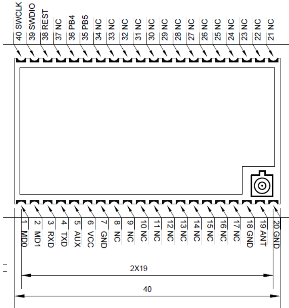
引脚定义表
