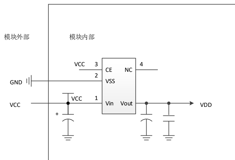
图 5-6 电源 LDO
