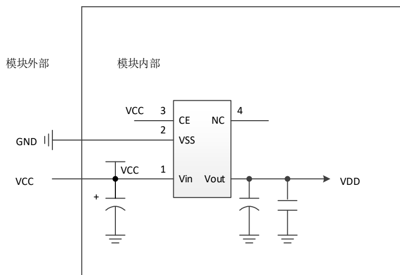
图 5-6 电源 LDO
