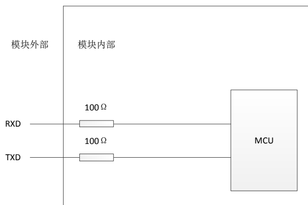
图 5-4 RXD、TXD 引脚内部结构示意图
