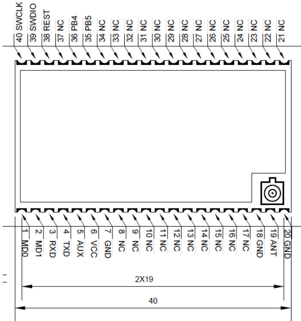
引脚定义表
