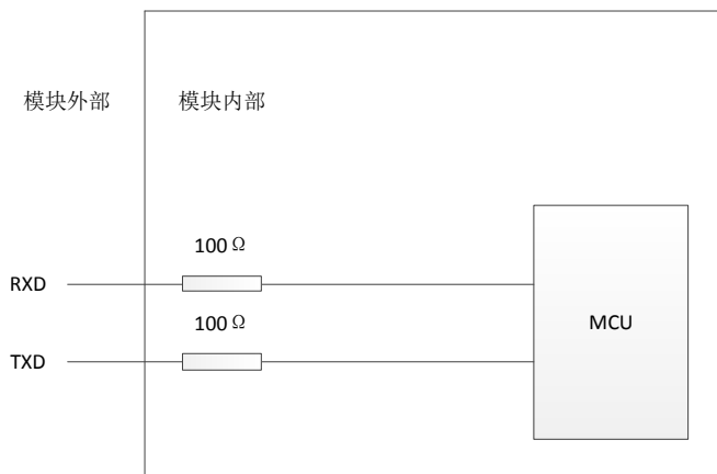
图 5-4 RXD、TXD 引脚内部结构示意图
