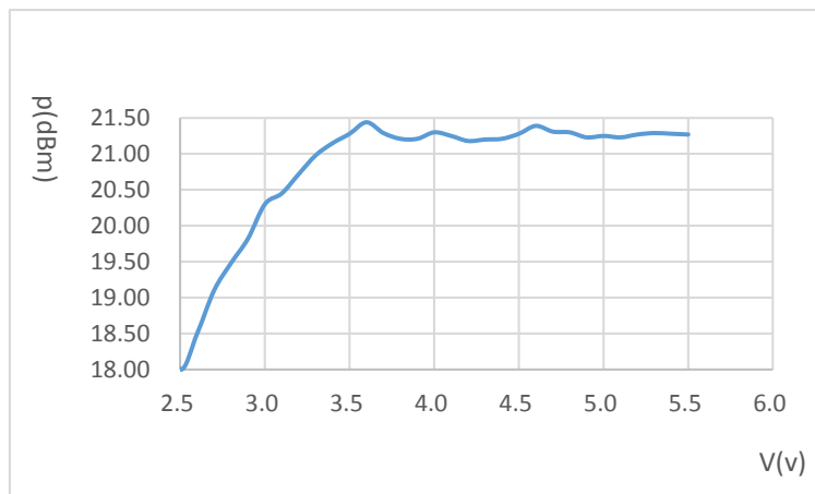
图 5-7 功率与电压的关系图
