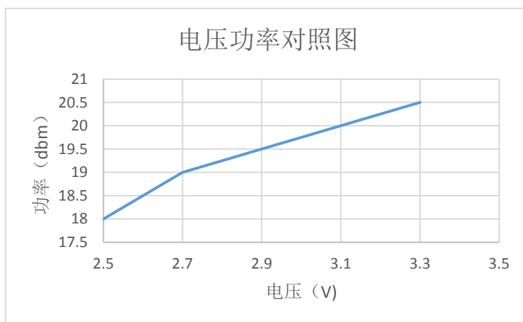
图 5-5 功率与电压的关系图
