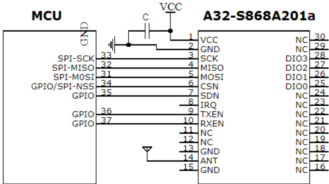
图 5-1 推荐连接图
