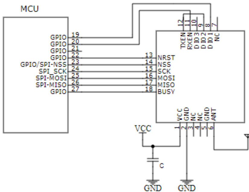
推荐连接图 2
