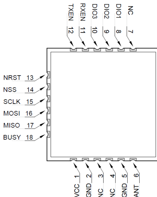
引脚定义表
