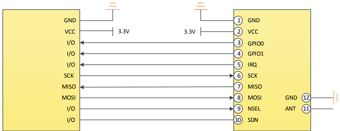
图 5-1 推荐连接图
