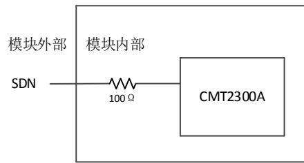
图 5-3 SDN 引脚局部连接示意图
