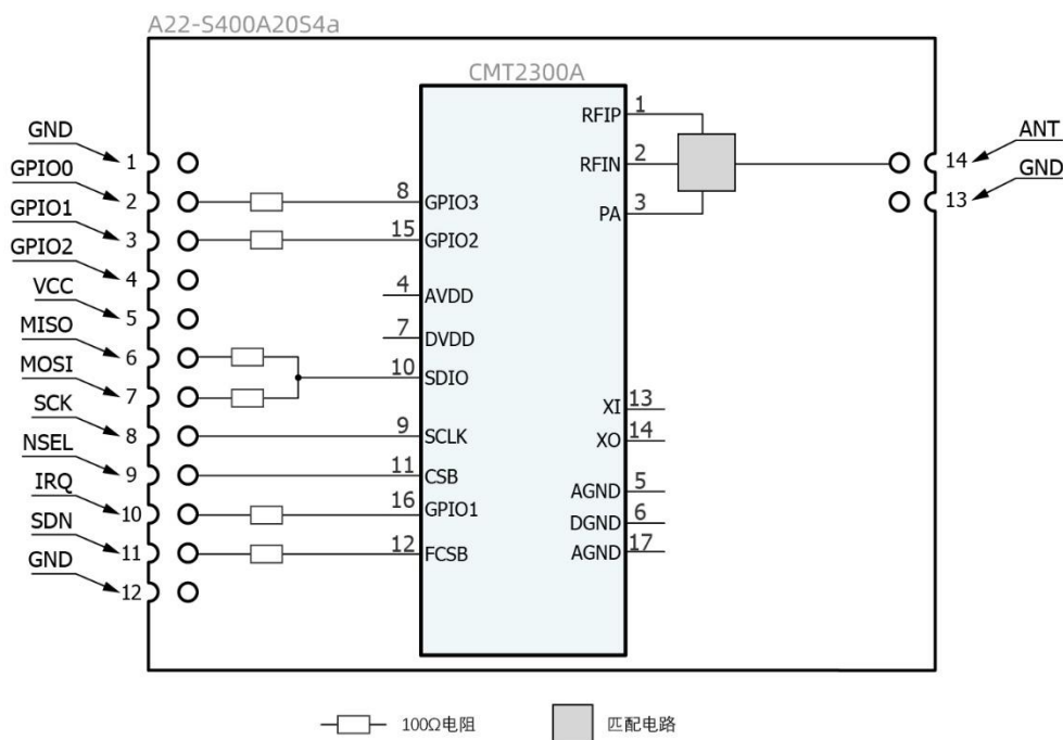
模块与芯片引脚对应关系图
