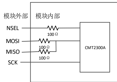
图 5-5 SPI 引脚局部连接示意图
