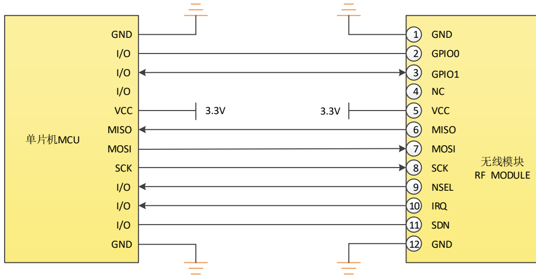
图 5-1 推荐连接图
