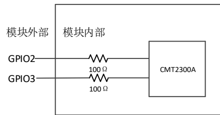
图 5-4 GPIO2、GPIO3 引脚局部连接示意图
