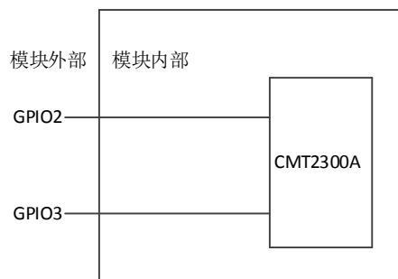
图 5-4 GPIO2、GPIO3 引脚局部连接示意图
