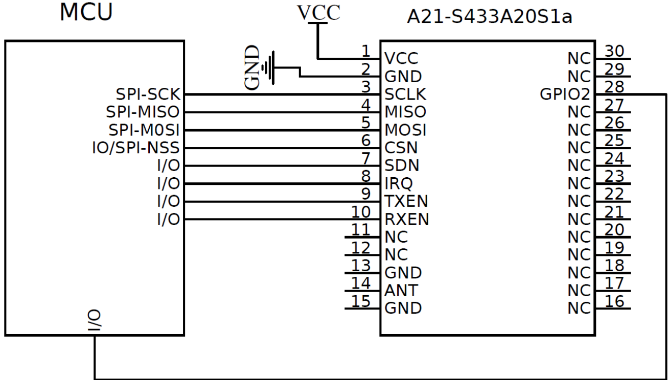
图 5-1 推荐连接图
