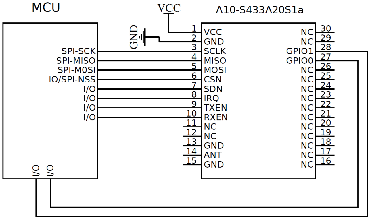
图 5-1 推荐连接图
