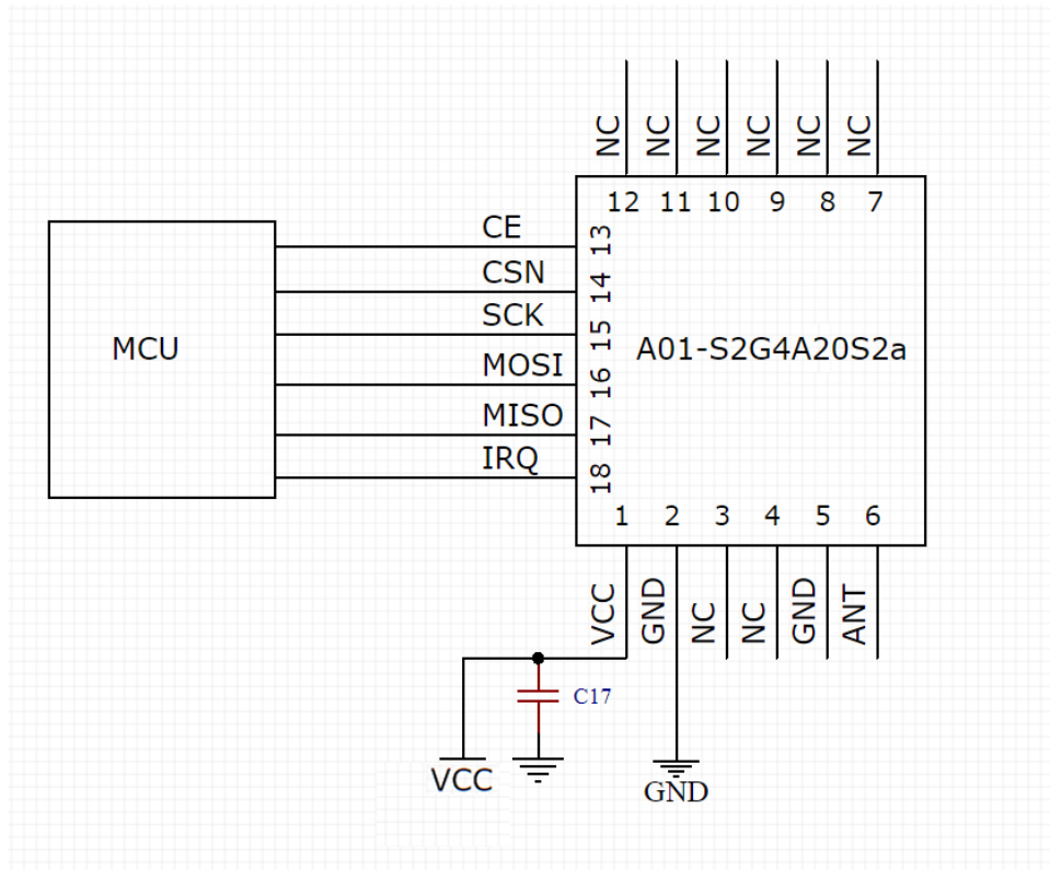
图 5-1 推荐连接图
