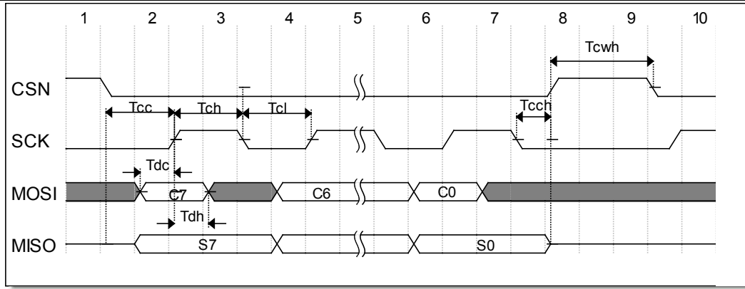
图 5-7 SPI 时序参考图
