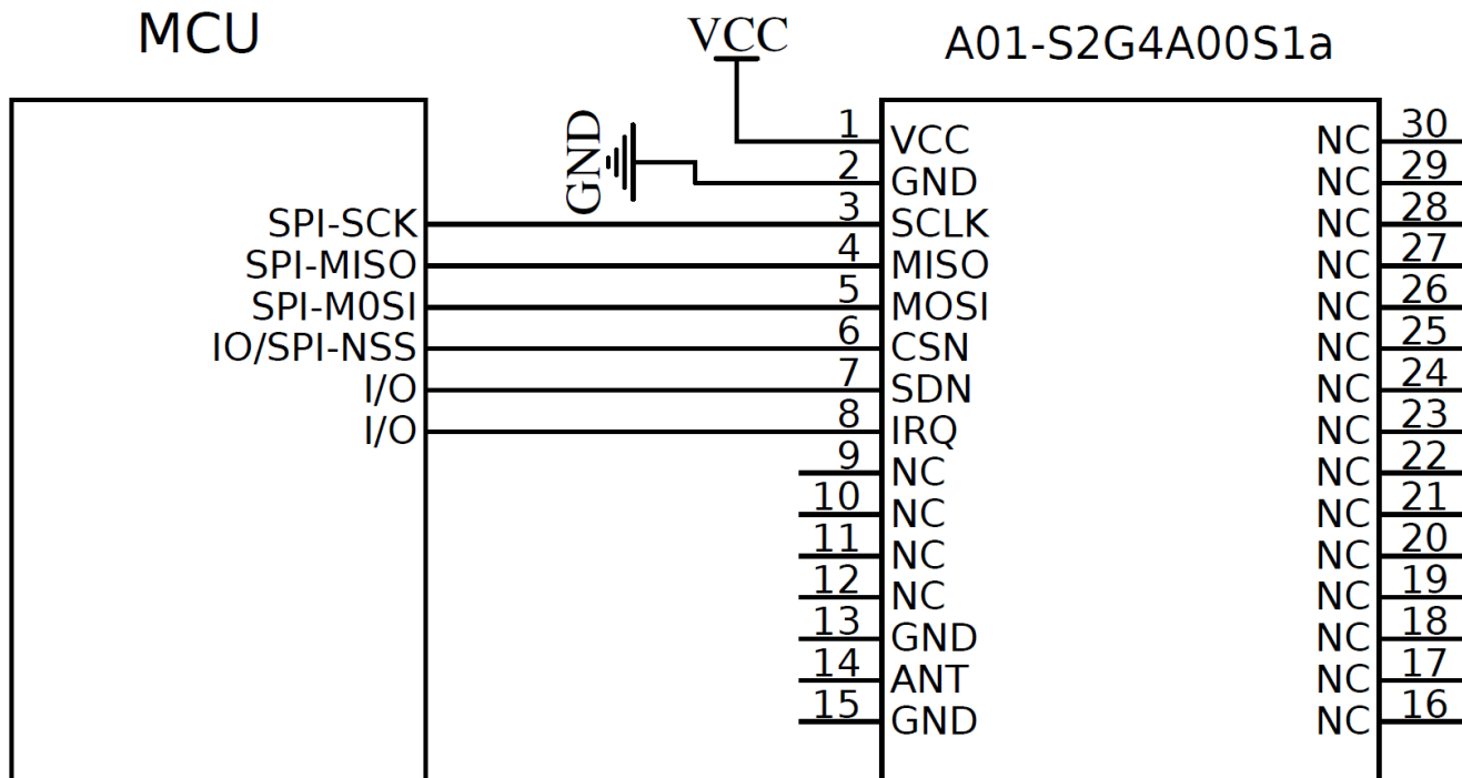
图 5-1 推荐连接图
